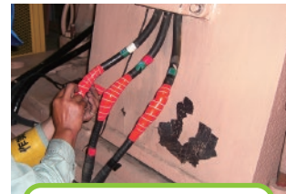
絶縁処理
